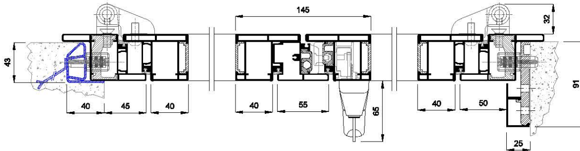
Sezione verticale
