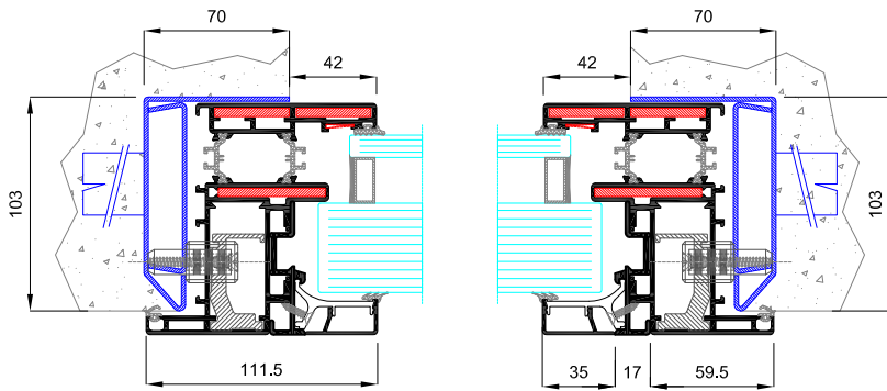
Sezione orizzontale fisso
