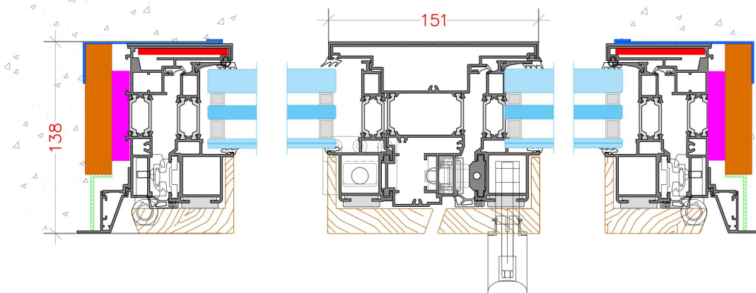
SEZIONE ORIZZONTALE A 2 ANTE Horizontal section with two doors
