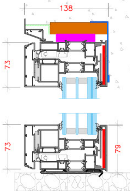
SEZIONE VERTICALE FINESTRA Longitudinal section Window
