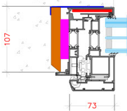
SEZIONE ORIZZONTALE A 2 ANTE Horizontal section with two doors
