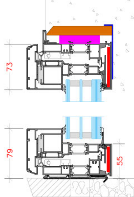
SEZIONE VERTICALE PORTAFINESTRA Longitudinal section Door
