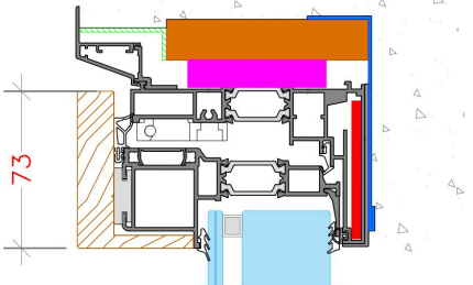
SEZIONE VERTICALE FINESTRA Longitudinal section Window
