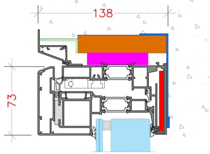
SEZIONE VERTICALE FINESTRA Longitudinal section Window
