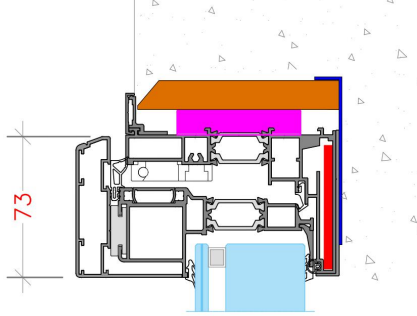
SEZIONE VERTICALE PORTAFINESTRA Longitudinal section Door
