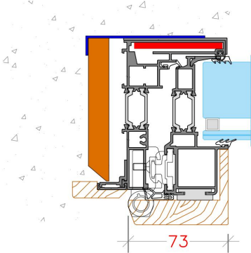
NODO LATERALE- LATO CERNIERA Lateral section- hinge side
