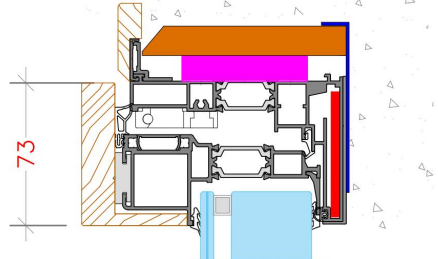
SEZIONE VERTICALE PORTAFINESTRA Longitudinal section Door
