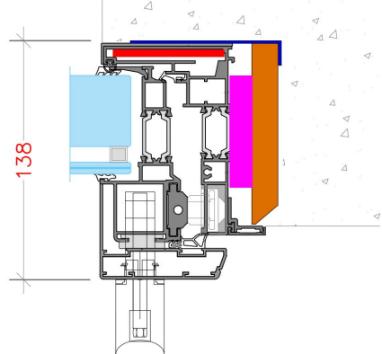
SEZIONE ORIZZONTALE A 2 ANTE Horizontal section with two doors
