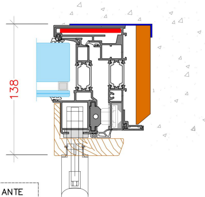
NODO LATERALE-LATO SERRATURA Lateral section-Lock side
